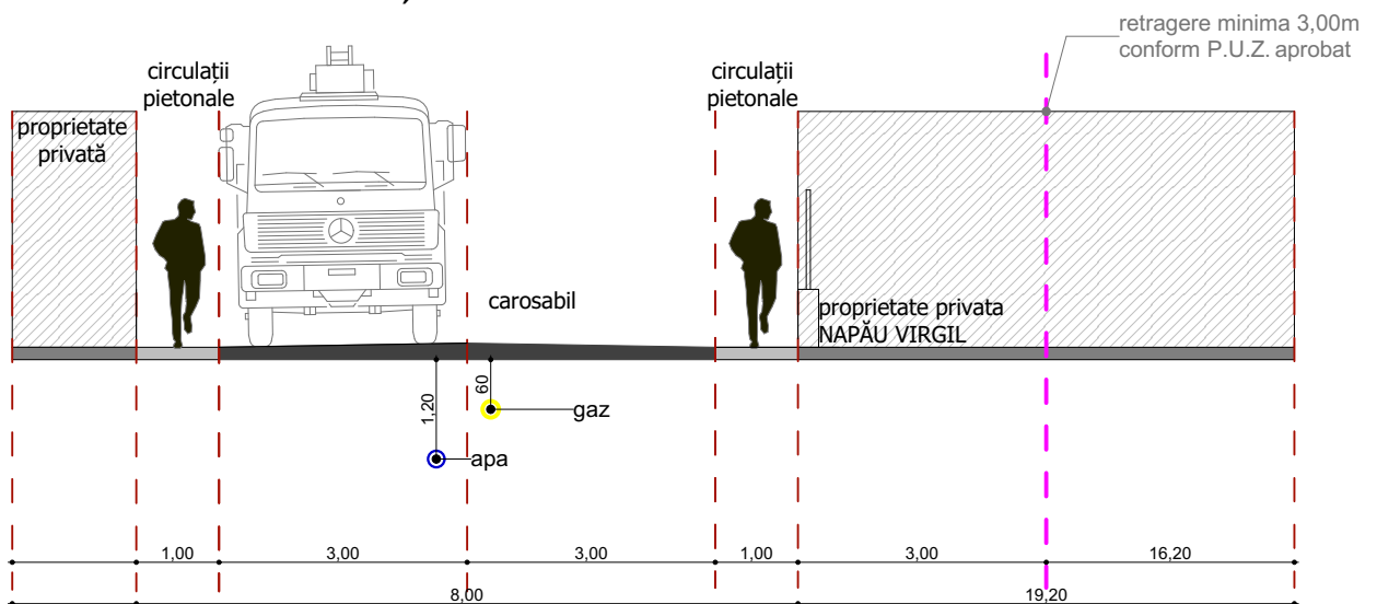
STR. FĂGĂRAȘ - 8 m profil transversal conform P.U.Z. aprobat
